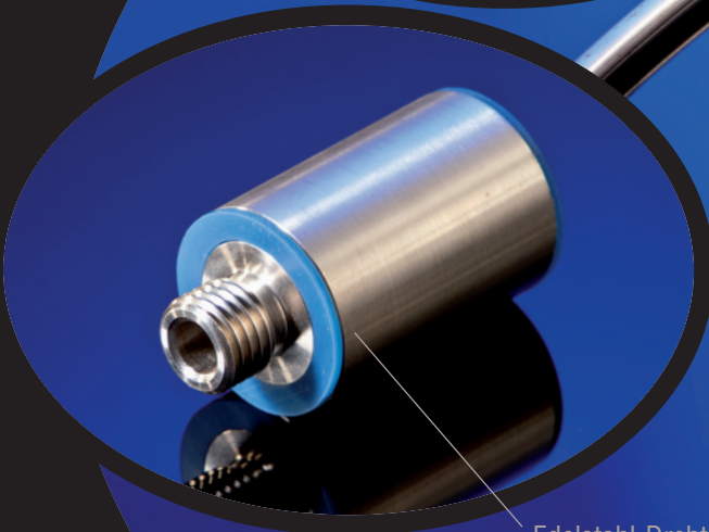
Edelstahl-Drehteil mit Silikon-Dichtung für Schalt- schränke der Hygieneindustrie
